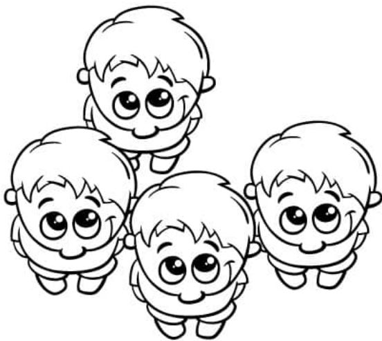
QUADRUPLETS
